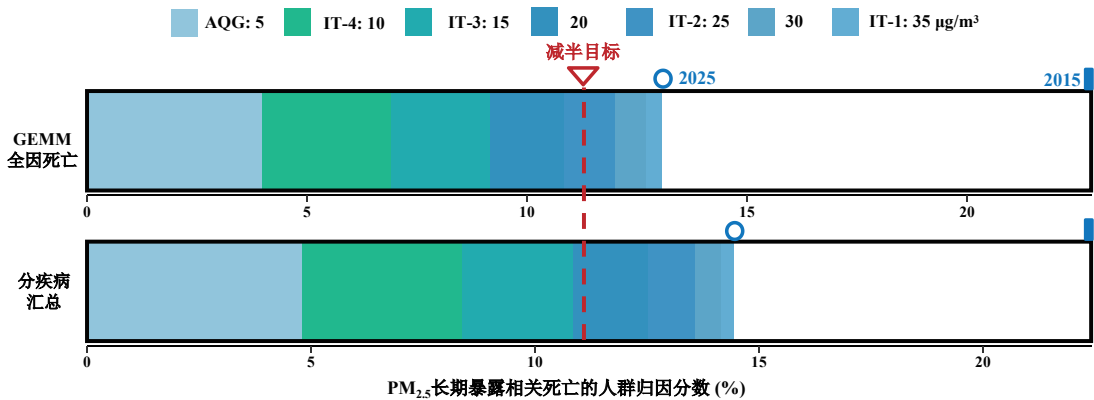
图 6.1 不同 PM 2.5 年均浓度限值对 WHO 减半目标总体实现进程的影响
