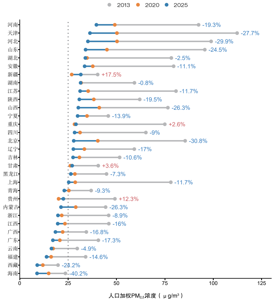
2013、2020 和 2025 年各省份人口加权 PM 2.5 浓度变化
