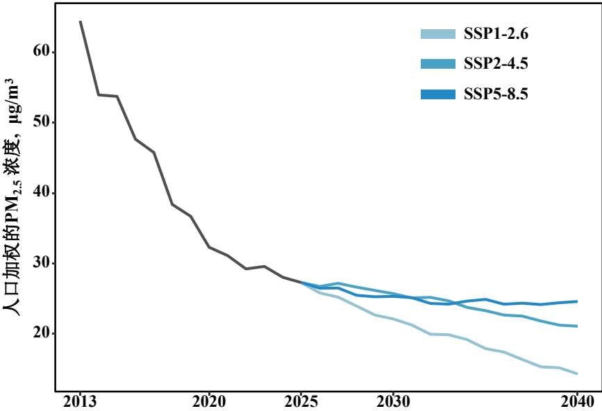
图 3.2 2013—2040 年三种政策情景下我国人口加权 \text{PM}_{2.5} 浓度的变化
