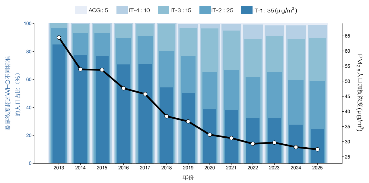
图 3.1 2013—2025 年我国人口加权 PM 2.5 浓度变化
